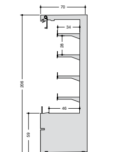
EI700-S
